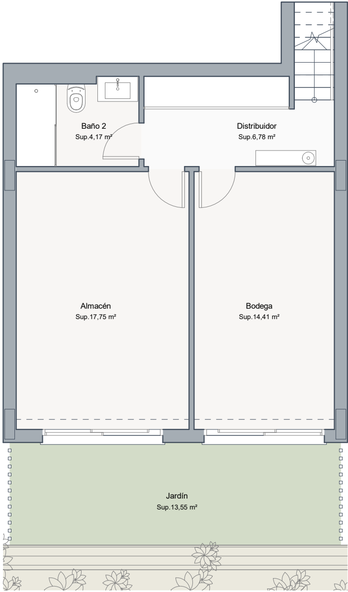
PLANTA SÓTANO
